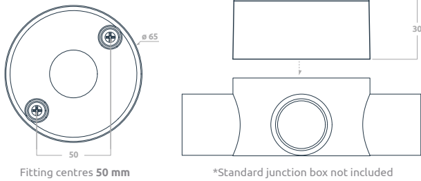
Conduit mount
